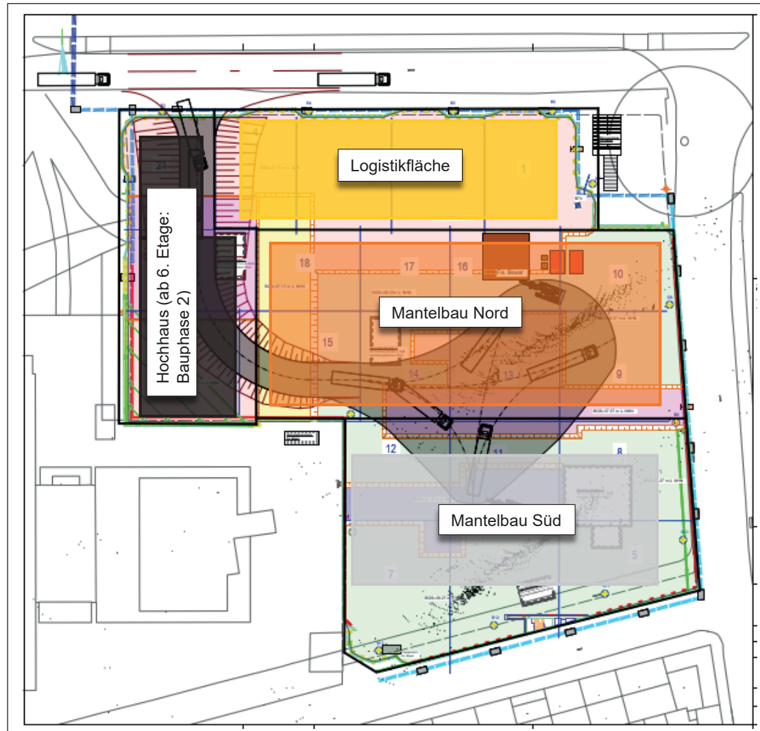
Übersicht Rohbaumaßnahme
